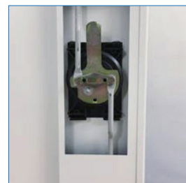
Triple bloqueo puertas
