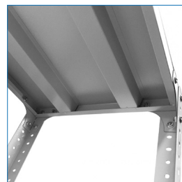
Bandeja con doble reforzamiento tipo omega
