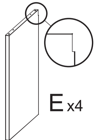
Placa vertical inferior (larga)
