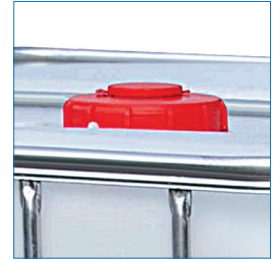
Tapa de llenado DN 150 con vente de HDPE de alta densidad con sello de anillo de EPDM
